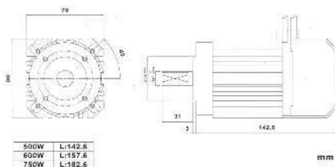
Motor / 馬達
